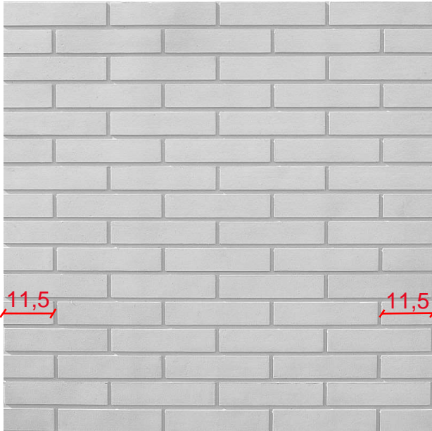
(C47 = 13 volle bakstenen x 93 rijen)
